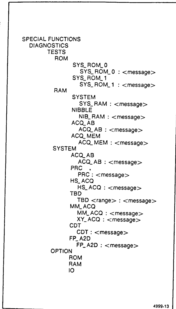
Figure 6-4. Diagnostic Menu.
